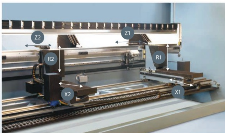
CNC опции заднего упора X1 - X2, R1 - R2, Z1 - Z2
